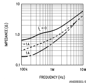
b) Output Impedance
